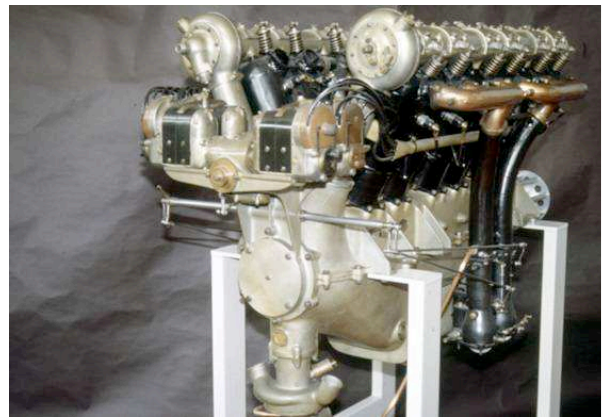
Moteur Renault refroidi par eau homologué en 1917, en service en 1918 (Breguet XIV). 12 cylindres en V, 22,10 L, 305 CV à 1550 tr/mm, 380 kg. ⇨
