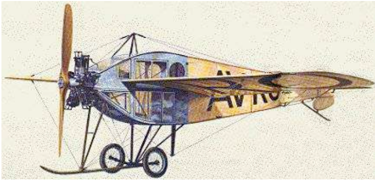
AVROF - A.V. ROE (1912) Premier monoplan fermé, par une structure en tubes d'acier couverte de toile et d'aluminium, et des fenêtres en cellulöid ↗
