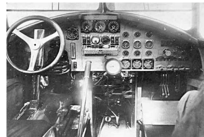
↑ Tableau de bord de l' "Arc en Ciel"
