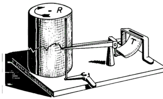
Thermomètre enregistreur à lame bimétallique
