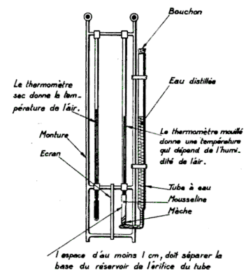
Psychromètre.
