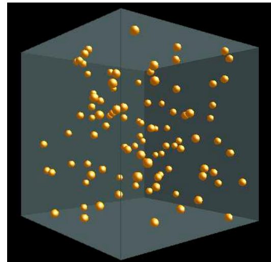
Simulation du mouvement désordonné des molécules d'un gaz (logiciel Modmol).
