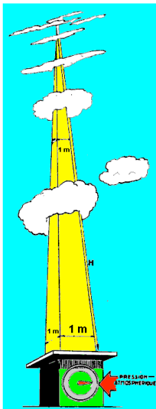
Pression = colonne d'atmosphère de 1 m 2
