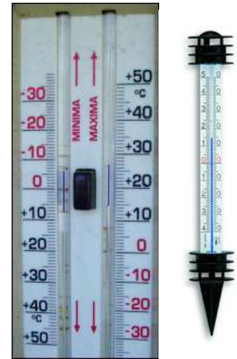
Thermomètre mini / maxi
